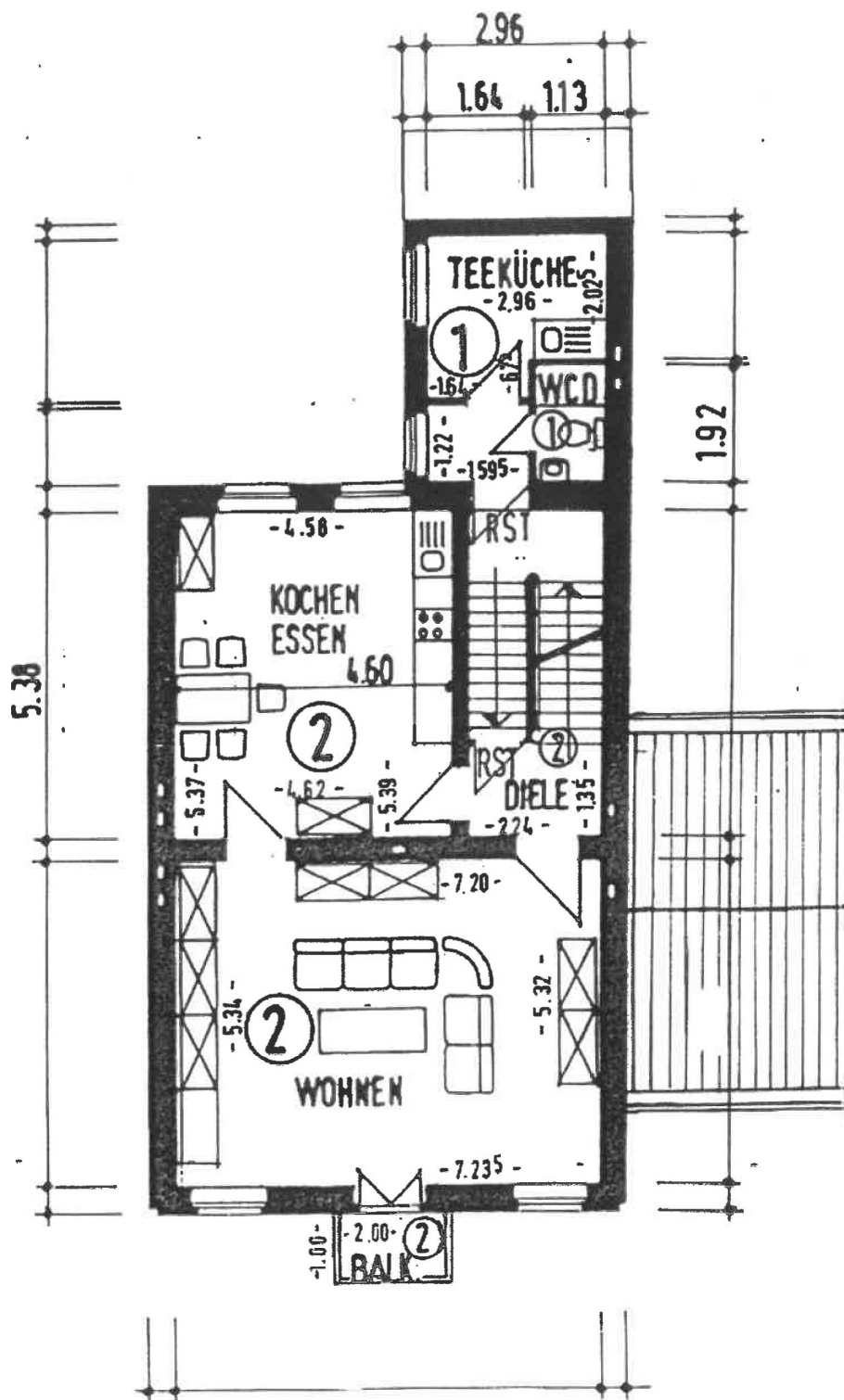
1. OBERGESCHOSS
